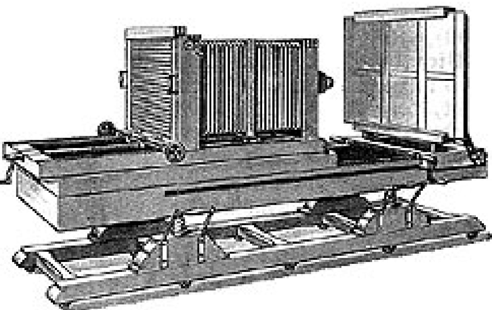
Fig. 8. Schwingcamera von Zeiss und Berner.
